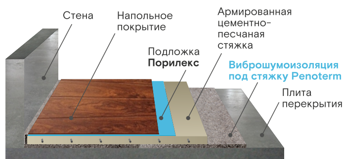
Конструкция плавающего пола под стяжку
